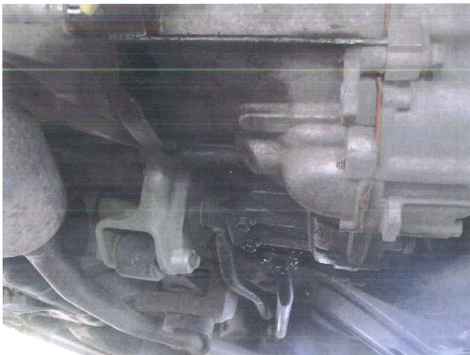
Bild 14 : Motor Ölverlust
